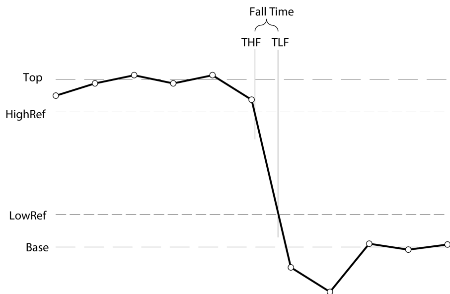
図2: 立下り時間
