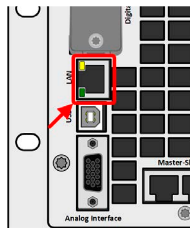
Bild 8 - LAN-Port
