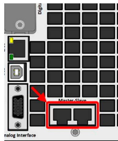
Bild 7 - Master-Slave-Busanschlüsse
