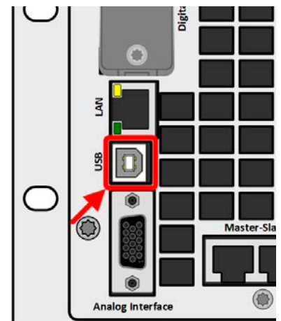
Bild 2 - USB-Anschluß
