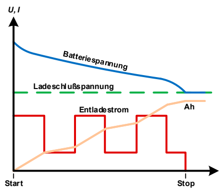
Dynamische Entladung
