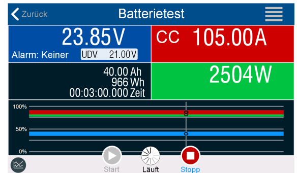
Bild 3 - Anzeigebispiel vom statischen Entladen
