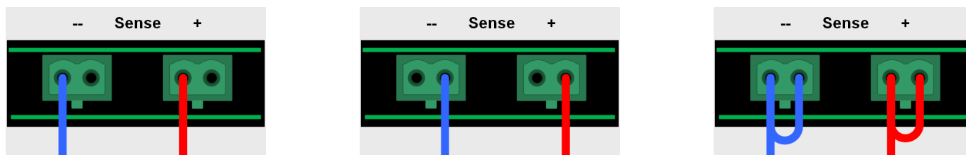
Figure 13 - Exemple de câblage de mesure à distance (bornier DC et Sense couvrent la voie de gauche à des fin d'illustration)
