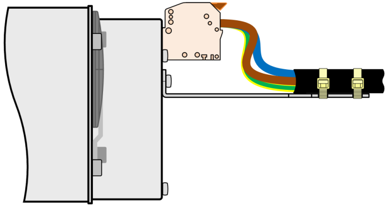
Figure 11 - Exemple de soulagement de traction
