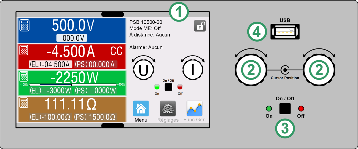
Figure 1 - Panneau de contrôle (exemple d'un PSB 10000 2U)
