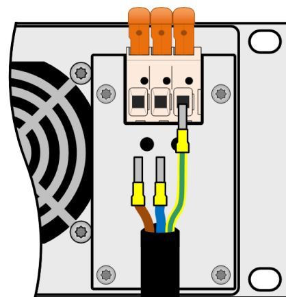
Figure 10 - Exemple de configuration câble AC
