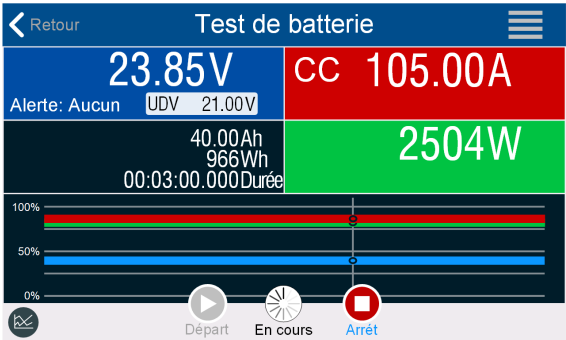
Figure 2 - Exemple de décharge statique
