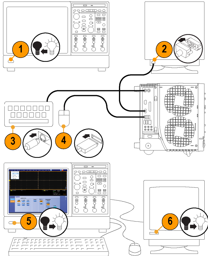
DPO7000C 系列
