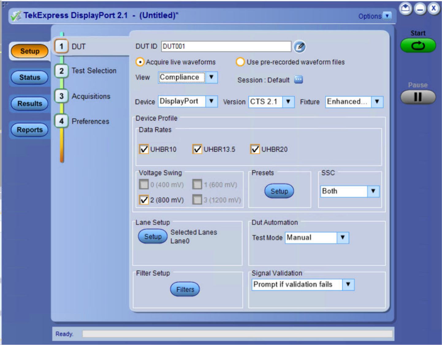
DUT panel
