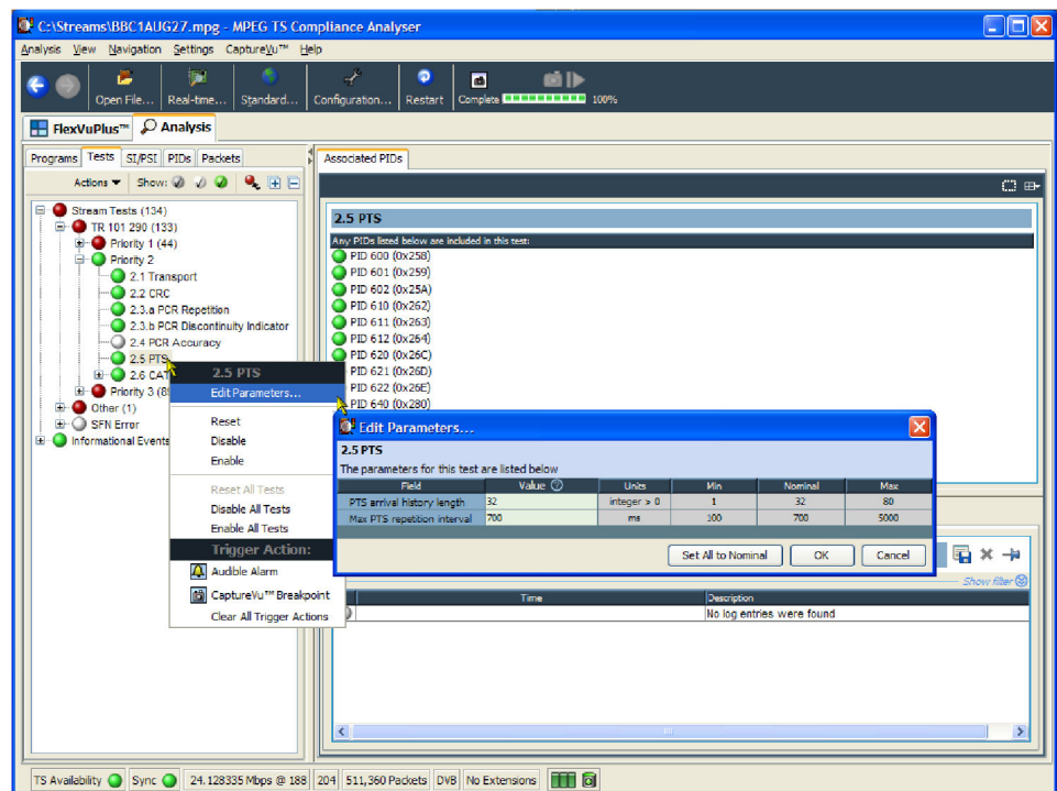
Figure 1-53: Test parameters
