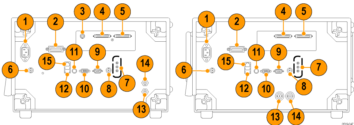
左図: RSA6100B シリーズ、右図: RSA5100A シリーズ
