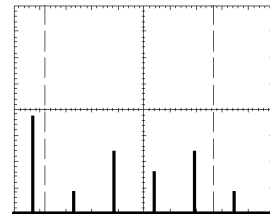
курсоры частоты
