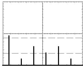
курсоры амплитуды
