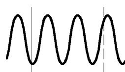
Курсоры времени
