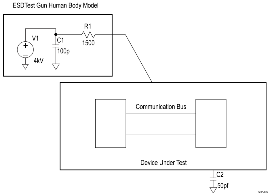
图 19: ESD 放电测试示例
