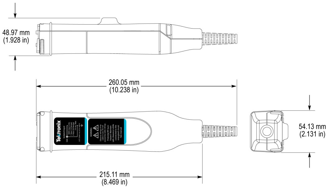
图 21: 传感器头部尺寸 (不带探头端部保护器)
