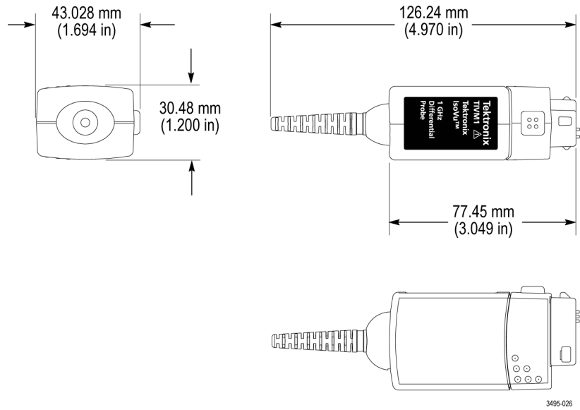
图 23: 补偿盒尺寸
