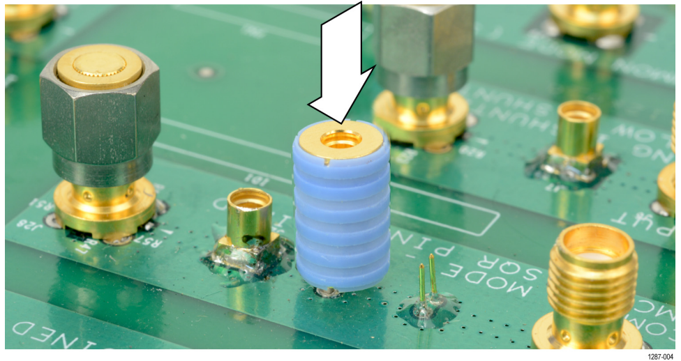
图 32: 将 MMCX 到 0.1 英寸 ( 2.54 毫米 ) 适配器按入合适位置
