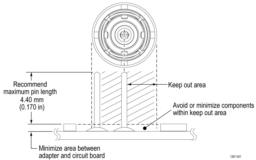
图 33: 适配器间隙要求
