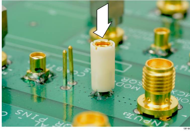
图 31: 将 MMCX 到 0.062 英寸 ( 1.57 毫米 ) 适配器按入合适位置
