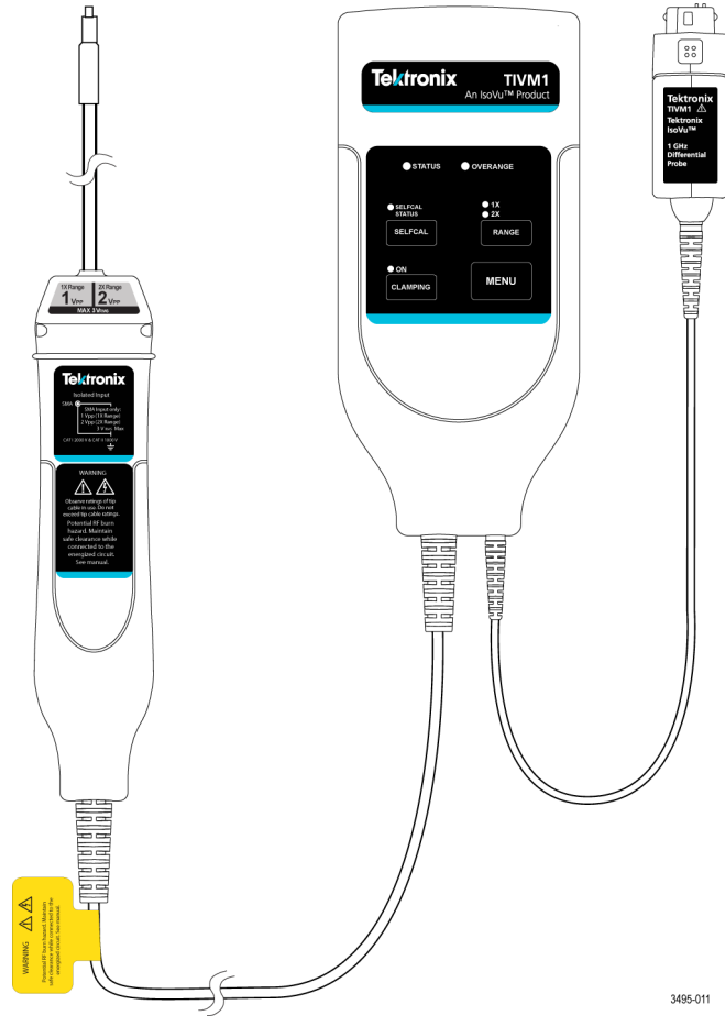
图 i: TIVM 系列 IsoVu 测量系统
