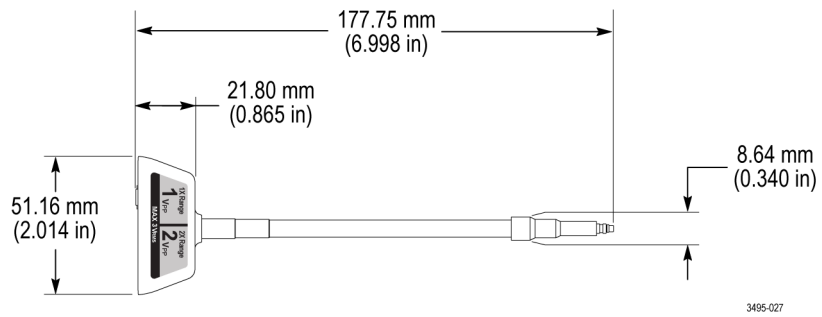
图 24: 探头端部适配器尺寸
