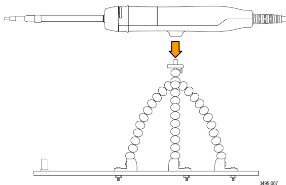
图 8: 将传感器头部连接到灵活三脚架
