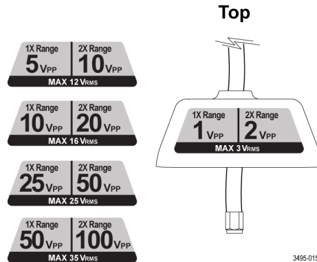
图 13: 上部传感器端部标签
