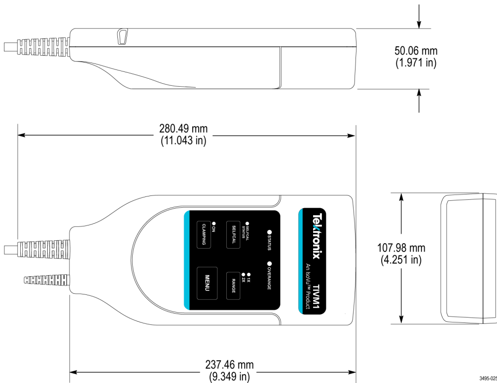
图 22: 控制器尺寸
