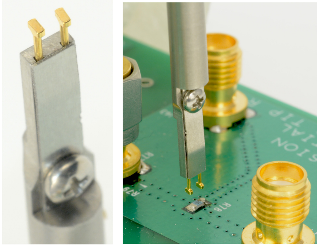
图 35: 使用焊接辅助件将方针安装到电路板
