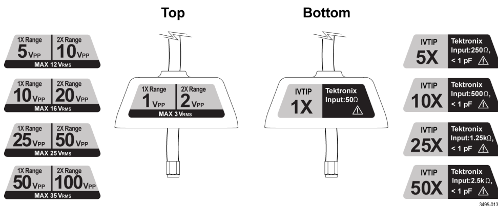
图 5: 传感器端部电缆上部和下部标签
