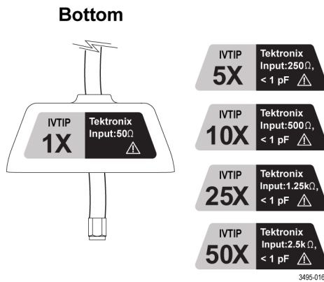
图 14: 下部传感器端部标签
