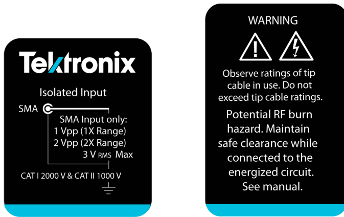
图 4: 传感器头部上的标签
