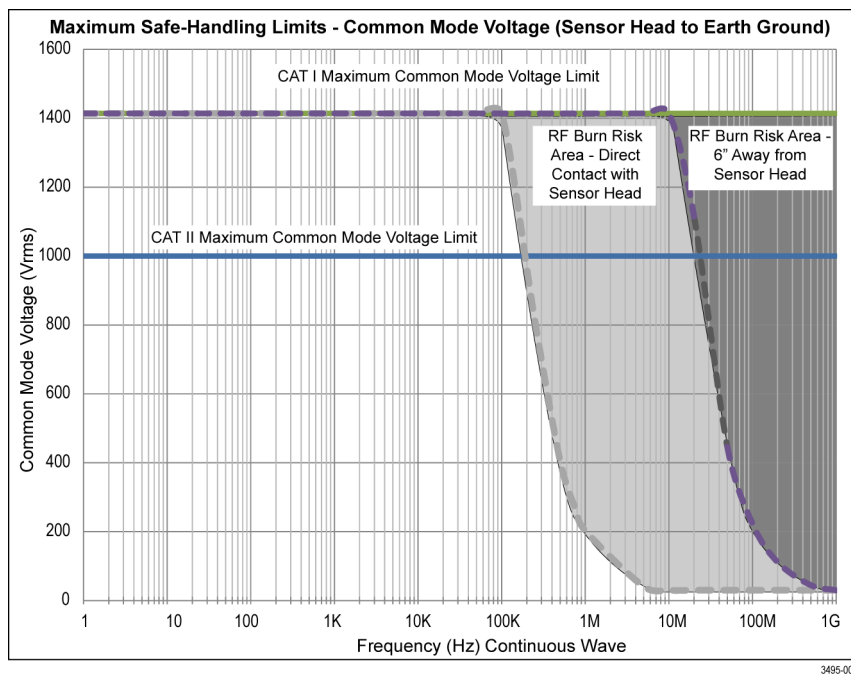
图 1: 传感器头部和接地之间共模电压的最大安全处理限制。
