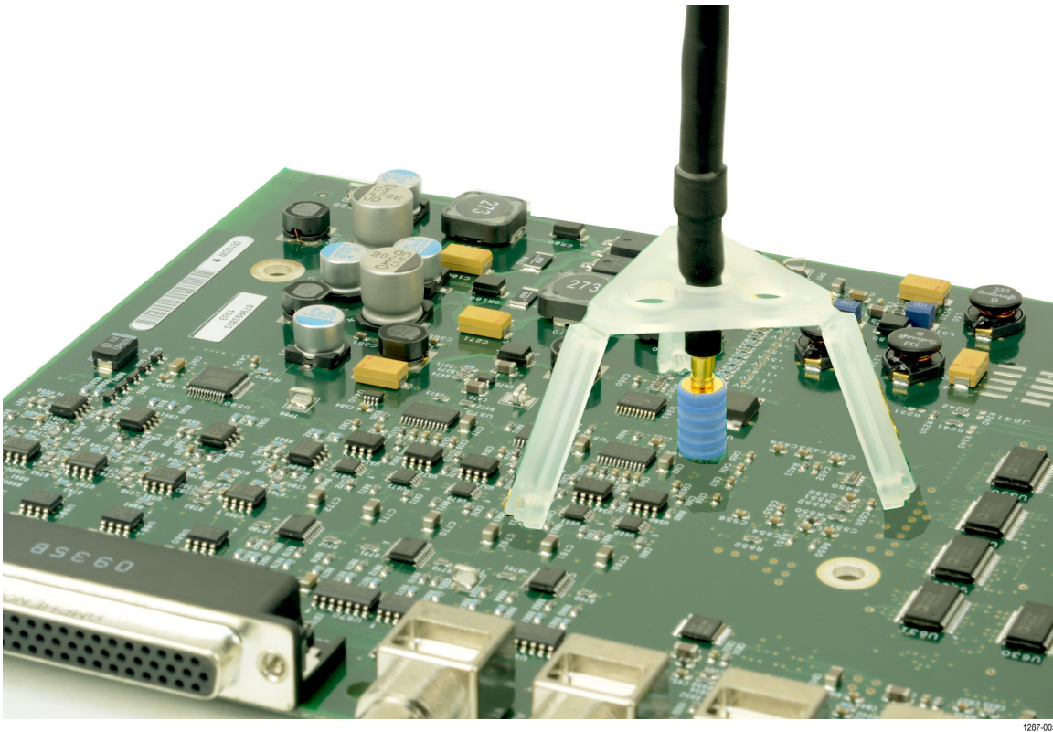
图 28: 将探头端部三脚架连接到电路板的适配器
