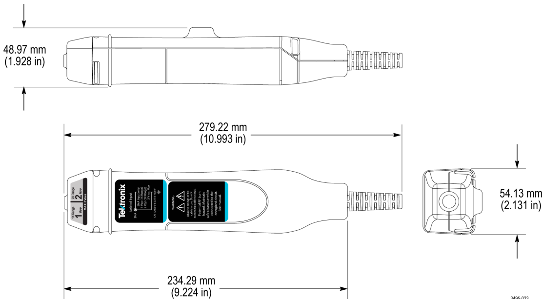
图 20: 传感器头部尺寸 (带探头端部保护器)
