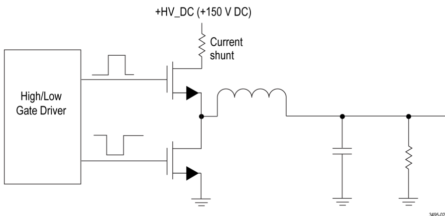
图 17: 高边电流分流器
