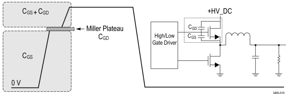
图 16: 高边导通特性
