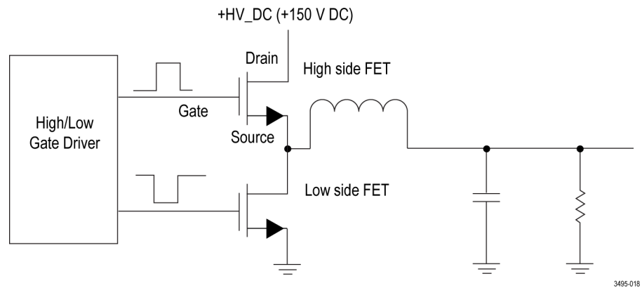
图 15: 半桥电路显示高边 FET 的选通、信号源和漏极
