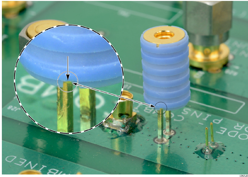
图 29: 对齐 MMCX 到 0.1 英寸 ( 2.54 毫米 ) 适配器与电路板
