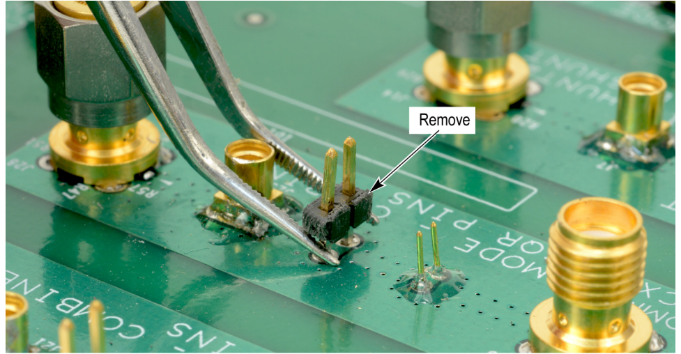
图 34: 移除电路板上方针的头部
