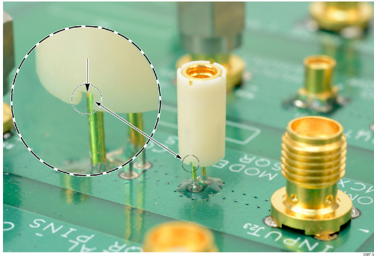
图 30: 对齐 MMCX 到 0.062 英寸 ( 1.57 毫米 ) 适配器与电路板
